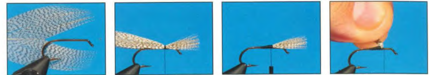
а) Подготовьте перо селезня, вырезав часть ости с бородками, оставшиеся бородки должны быть в 1,5 раза длиннее высоты крылышек. Отмерьте необходимую длину бородок в соответствии с размерами крючка и закрепите перо на цевье одним из способов, показанных на рис. 108, 109 или 112. Отрежьте излишки пера и переведите монтажную нить к месту первого закрепляющего витка.
