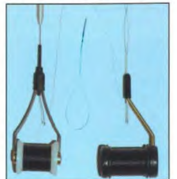
Рис. 95. Продеватели монтажной нити
