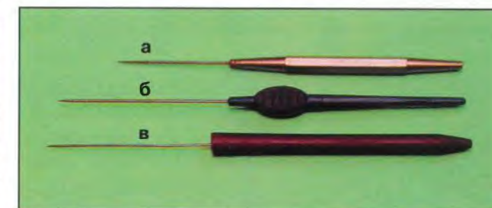
Рис. 54. Основные типы даббинговых игл
