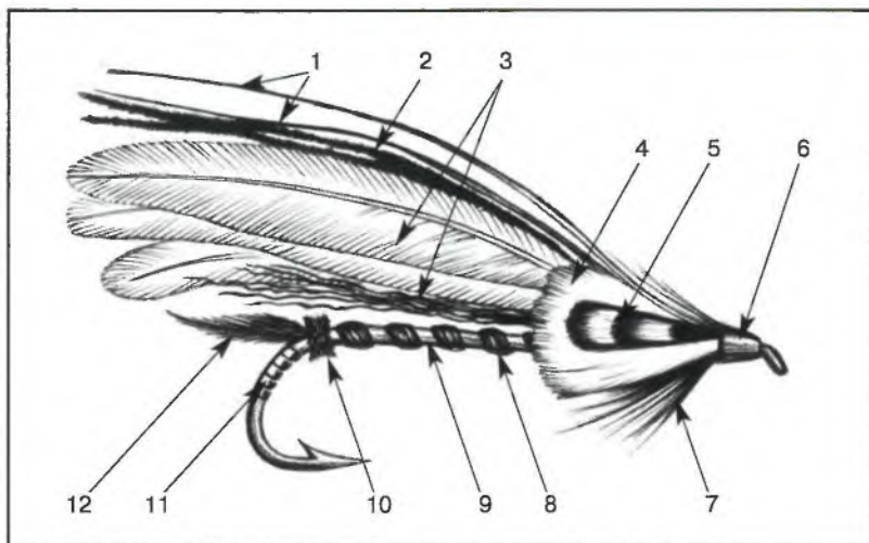
Рис. 172. Строение стримера
